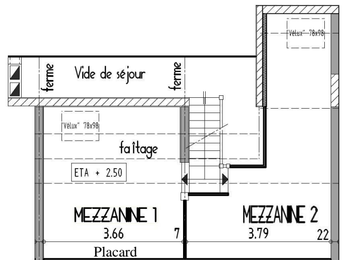
ETAGE
