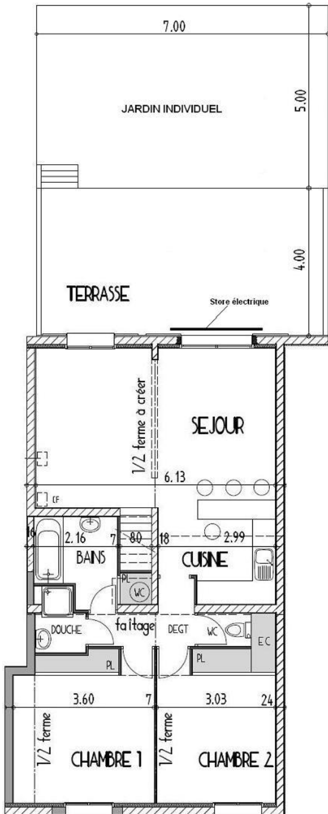
REZ-DE CHAUSSEE
