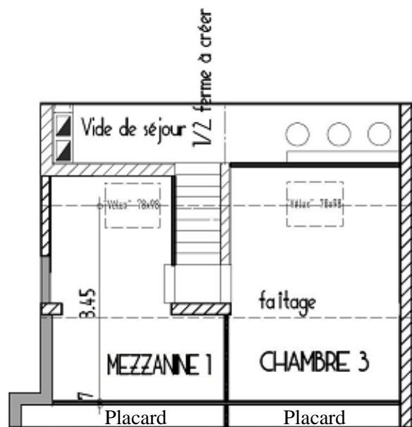
ETAGE
