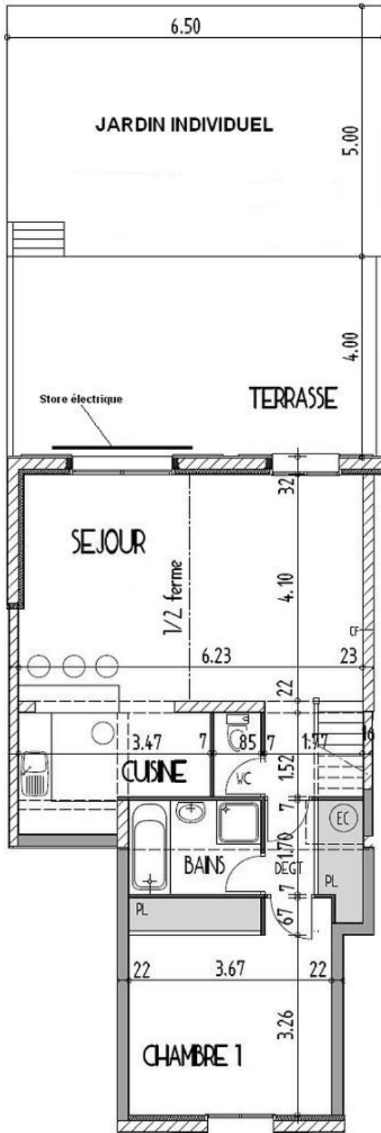
REZ-DE CHAUSSEE
