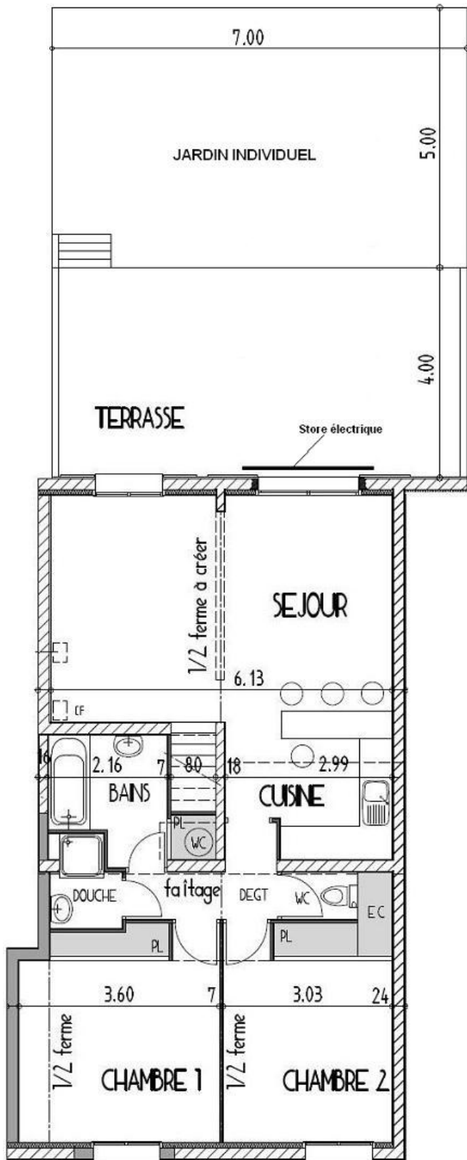
REZ-DE CHAUSSEE
