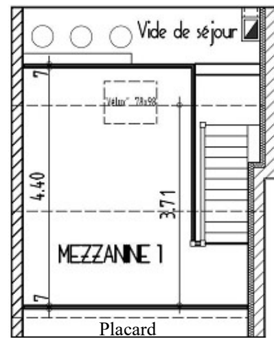
ETAGE
